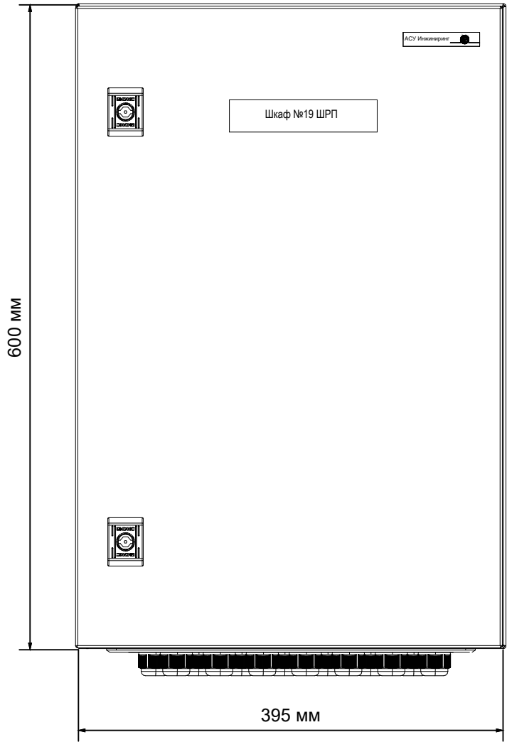
Вид спереди
