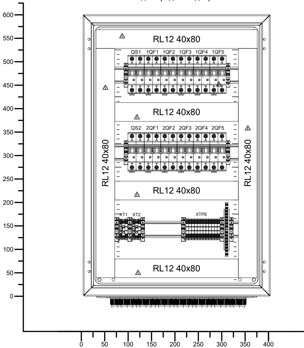
Вид спереди без дверей
